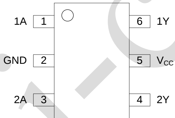
SOT363/SOT23-6
